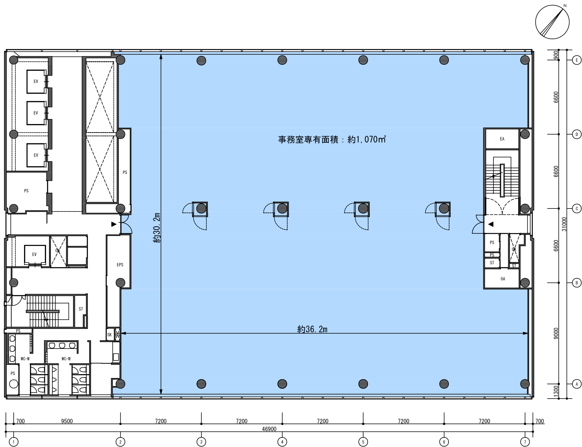
第二田町ビル 基準階平面図
