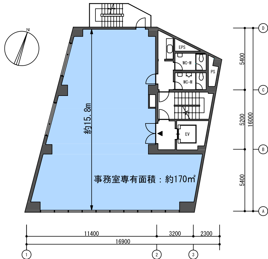
芝カンエスワカツビル 基準階平面図
